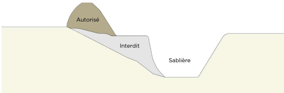
Figure 7. Nivellement autorisé et prohibé
