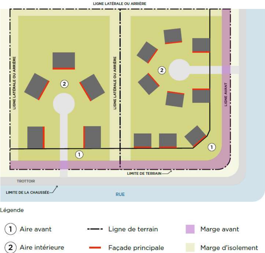
Figure 3. Figure 4. Délimitation des aires et des marges d'un projet intégré
