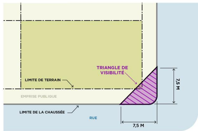
Figure 8. Triangle de visibilité
