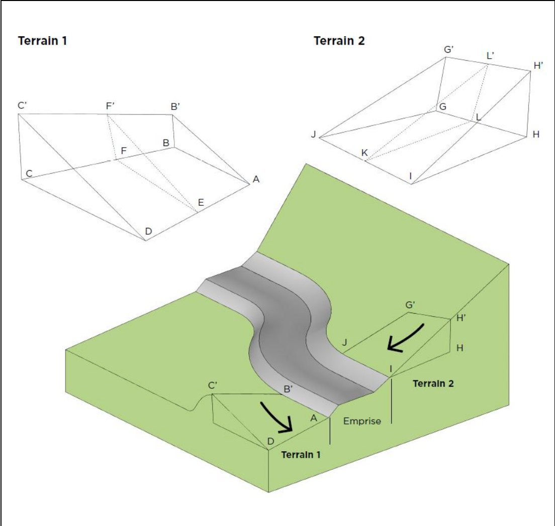
Figure 13. Calcul de la pente d'un terrain
