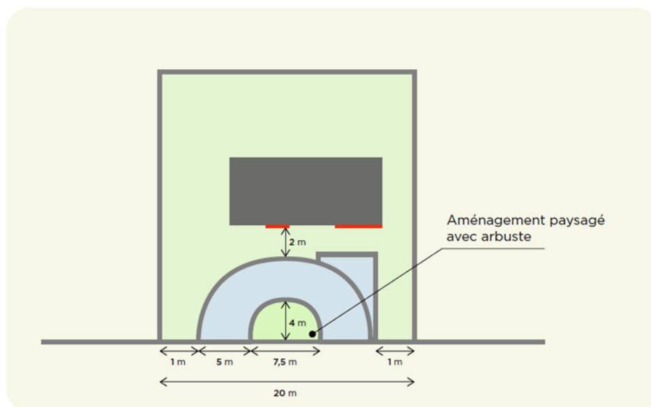
Figure 12. Aménagement d'une aire de stationnement en demi-cercle
