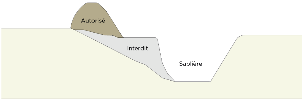
Figure 10. Nivellement autorisé et prohibé
